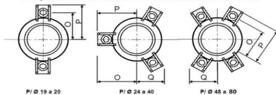
POSIÇÃO DOS GRAMPOS PARA BUCHA DE FLANGE EXTRA CURTA.
