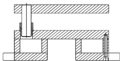
Com calços prolongadores
